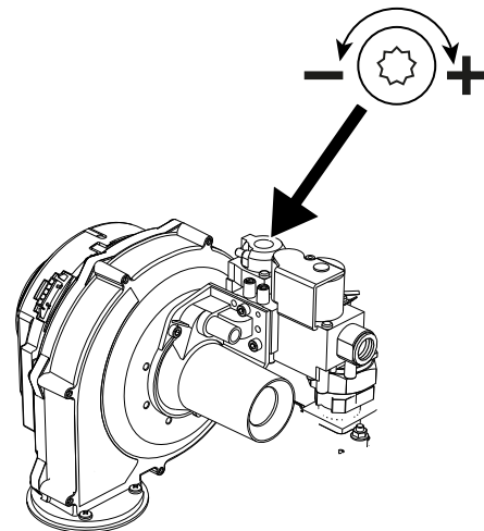
fig. 96 - Vite di regolazione della minima portata OFFSET
